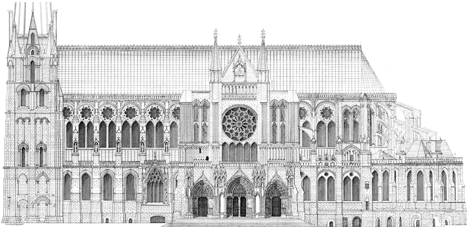
3. CHARTRES: KATHEDRALE. 1 : 400.
